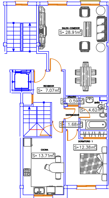
Planta primera
