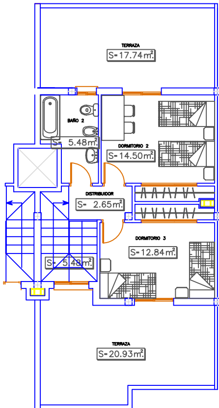
Planta ático
